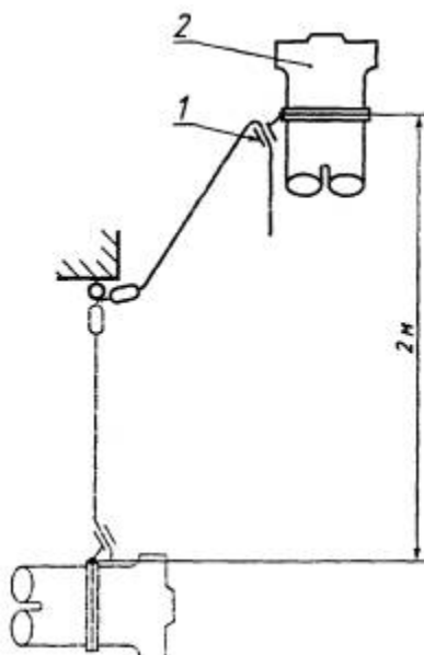
Рисунок 10 - Испытания динамических характеристик системы, состоящей из привязи, соединенной непосредственно с СИЗ от падения ползункового типа на гибком анкерном канате
