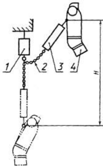
Рисунок 4 - Испытание динамических характеристик амортизатора в качестве компонента
