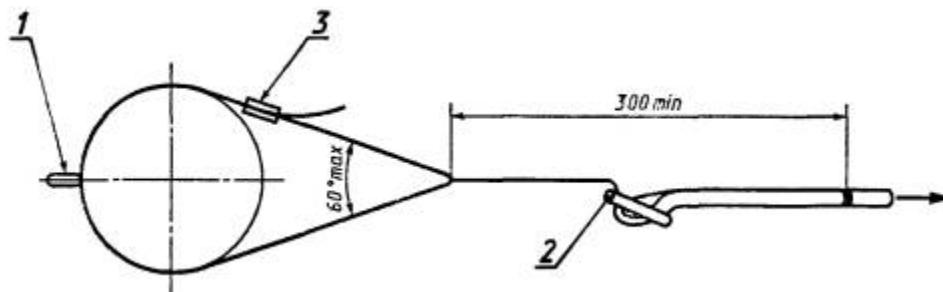
Рисунок 12 - Испытание статической нагрузкой удерживающей привязи
